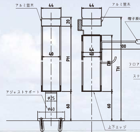
アジャストタイプ縦断面図
