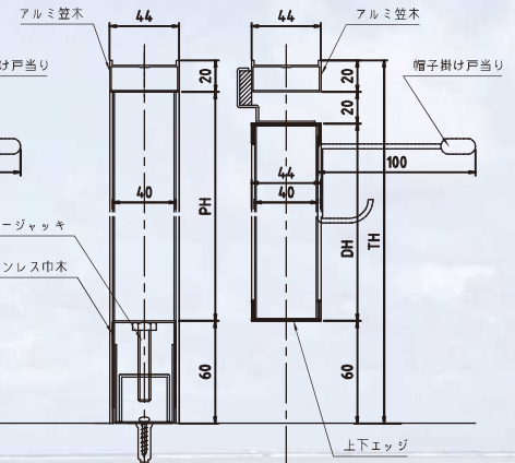
巾木タイプ縦断面図
